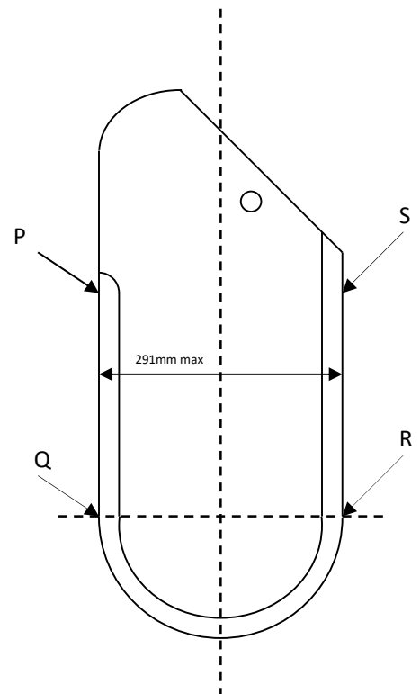
Rudder Blade
