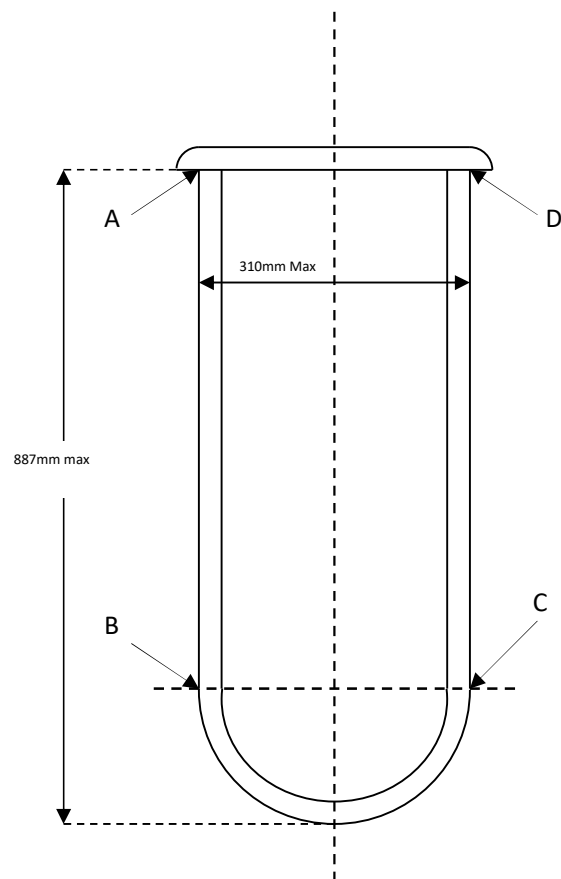
Daggerboard
